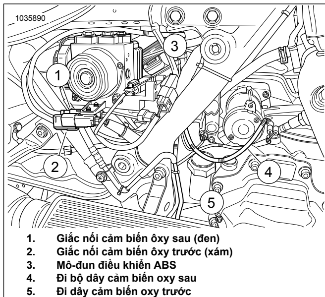
Hình 16. Đi bộ dây cảm biến của ATM
