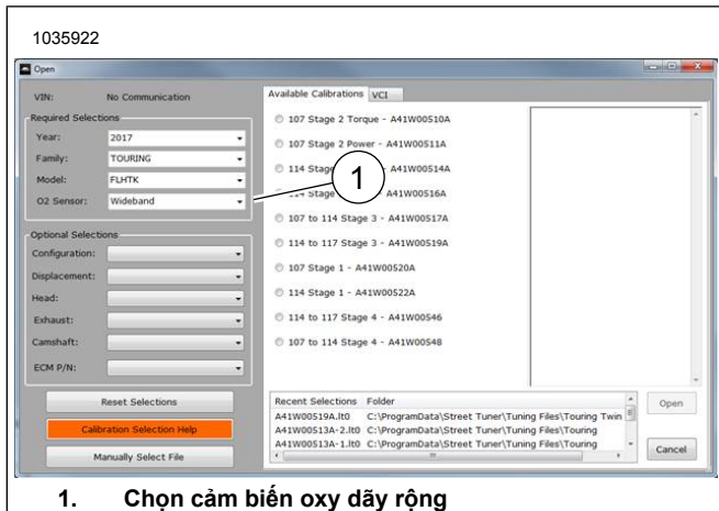
Hình 26. Chọn cảm biến oxy dây rộng
