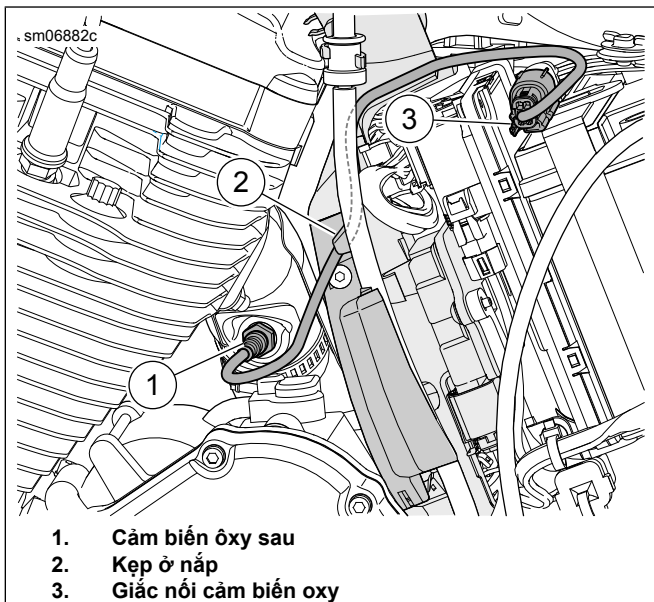
Hình 46. Cảm biến oxy sau
