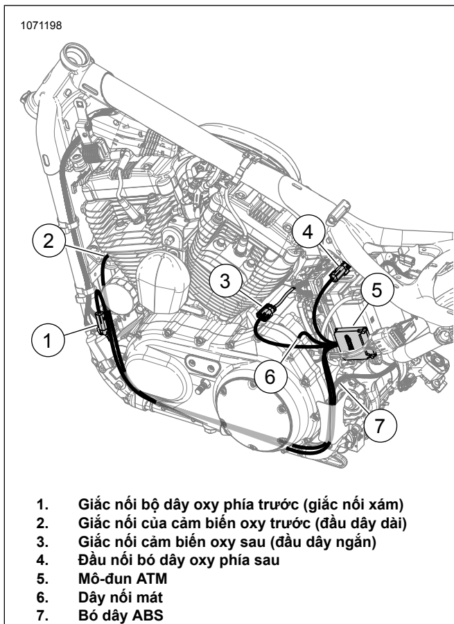
Hình 50. Đi bó dây ATM (chỗ chuẩn bị sẵn)
