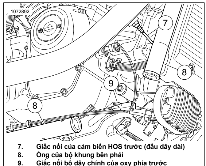
Hình 25. Đi bó dây phía trước của ATM (Tháo bớt phụ tùng để nhìn cho rõ)
