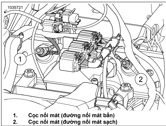
Hình 15. Vị trí cọc nối mát ở hộp ắc quy
