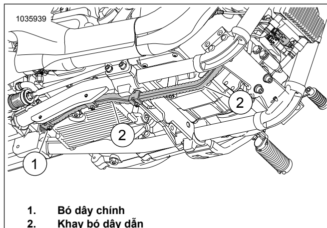
Hình 44. Khay bó dây dẫn
