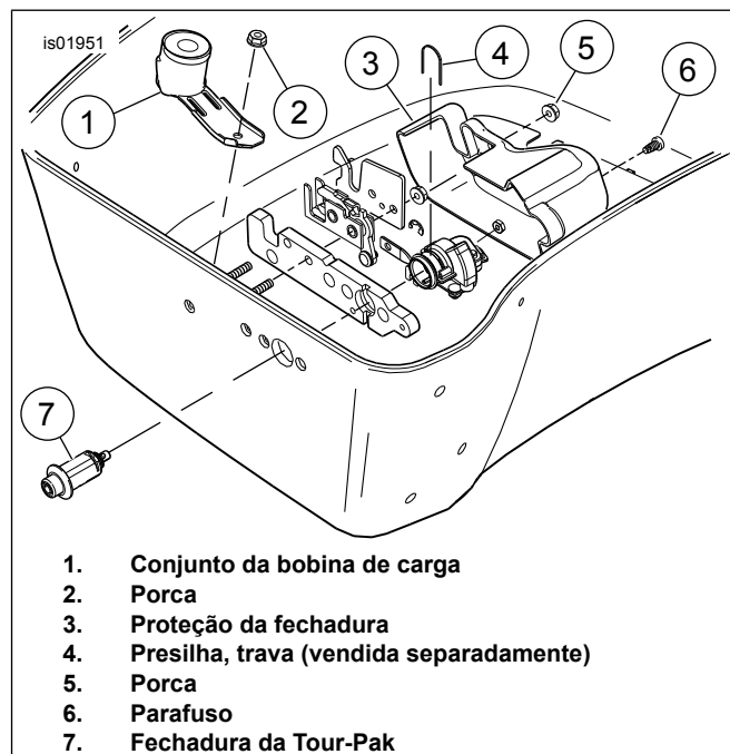
Figura 1. Instalação da bobina de carga da antena e da fechadura da Tour-Pak
