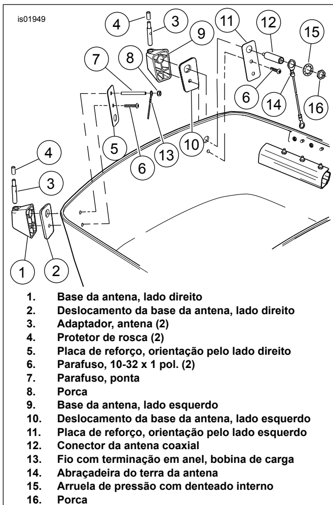
Figura 2. Instalação da base da antena
