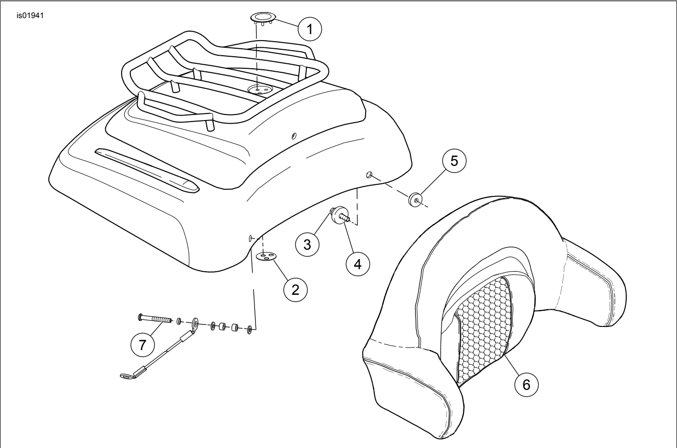
Figura 5. Peças de reposição para o kit de instalação da Tour-Pak (superior)
