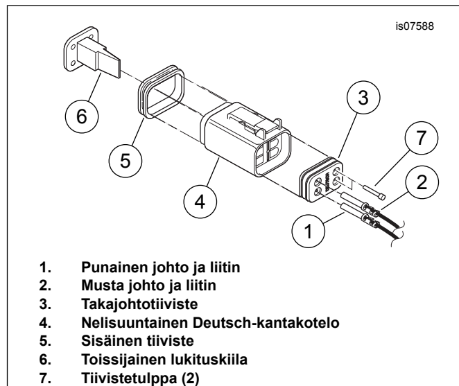
Kuva 2. Kiinnitä liittimet Deutsch-kantakoteloon
