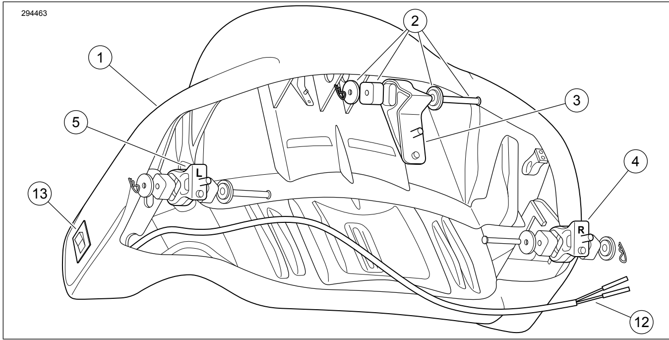
Kuva 4. Huolto-osat, King Tour-Pak -selkänöjasarjat 52300312, 52300314, 52300316, 52300317, 52300334, 52300574
