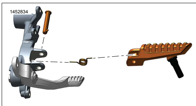
Figur 3. Fodhviler - fører - højre
