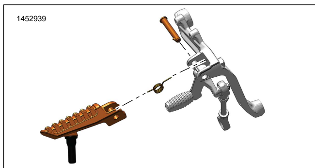
Figur 4. Fodhviler - fører - venstre
