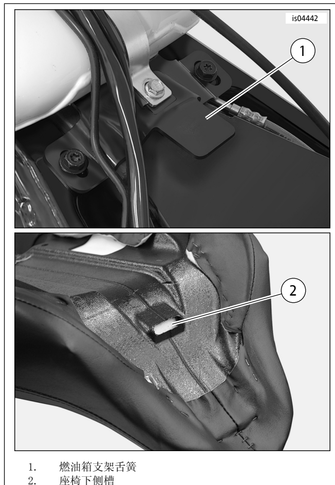
图1。座椅前底架
