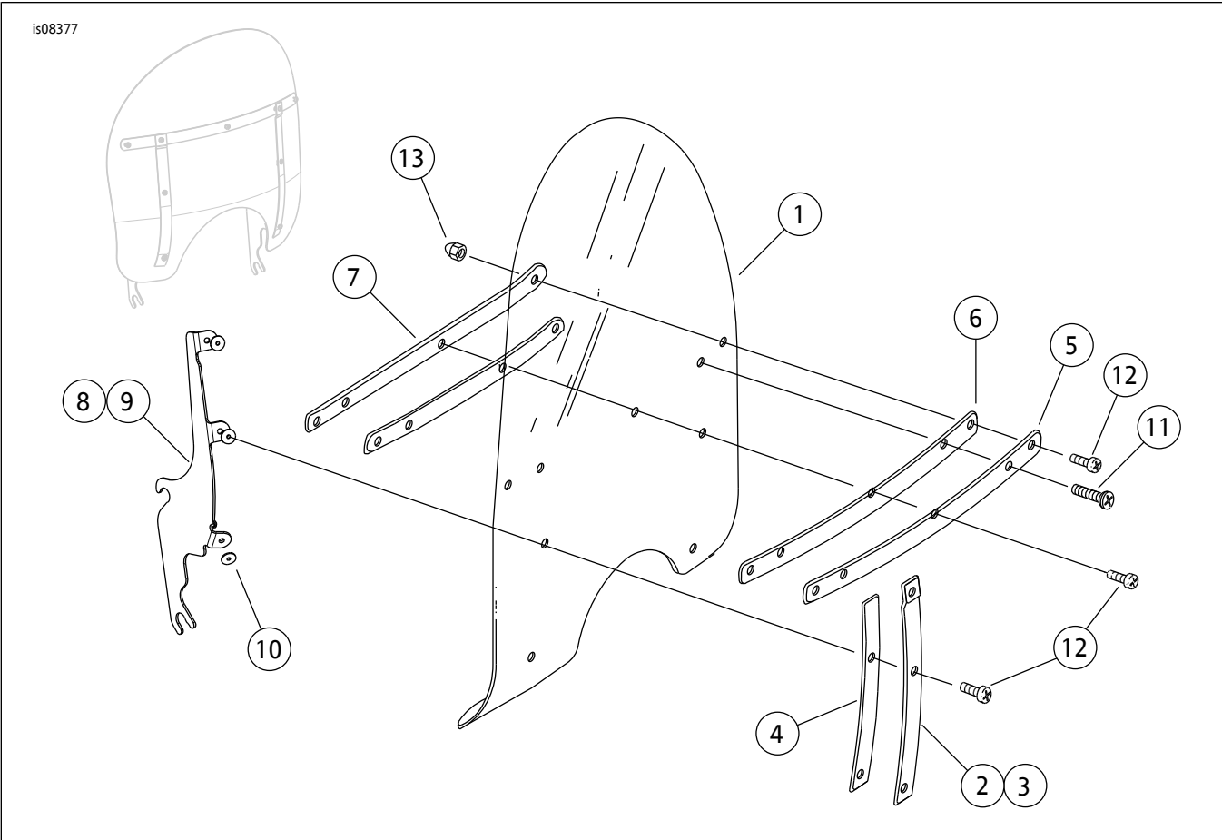
图1。套件内容：挡风玻璃（典型）
