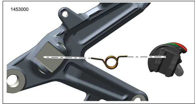
图5。回弹弹簧方向-右侧
