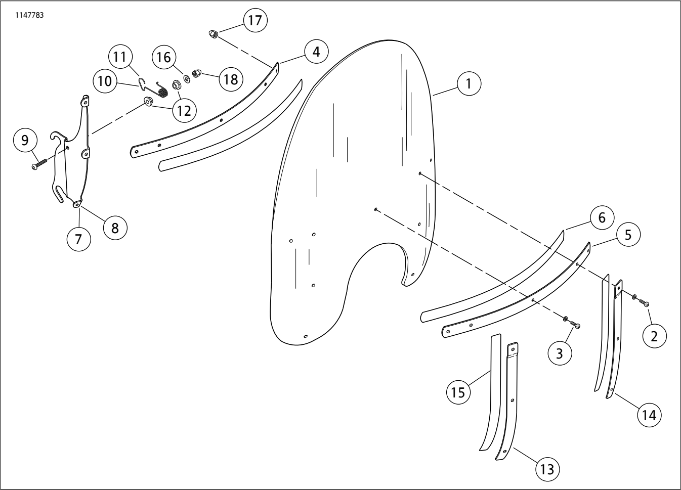
图1。维修零件：挡风玻璃组件
