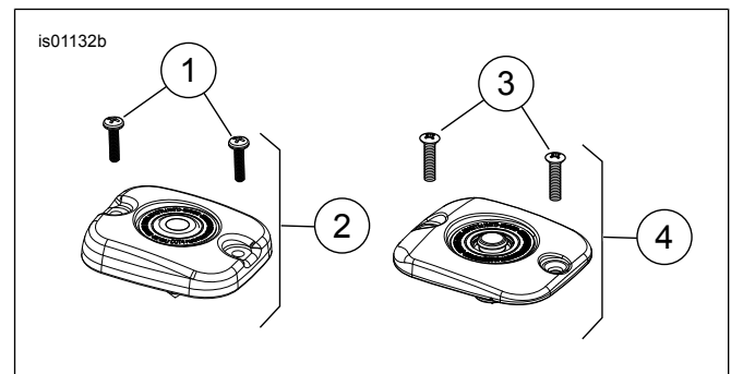
Abbildung 1. Ersatzteile: Hauptbrems-/Geberzylinderabdeckungssatz
