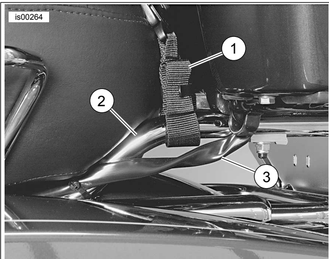
Abbildung 5. Quetschen der Kabelbäume vermeiden
