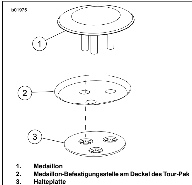
Abbildung 3. Anbringen des Medaillons
