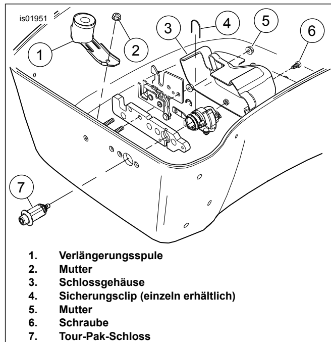
Abbildung 1. Einbau der Antennenverlängerungsspule und des Tour-Pak-Schlusses
