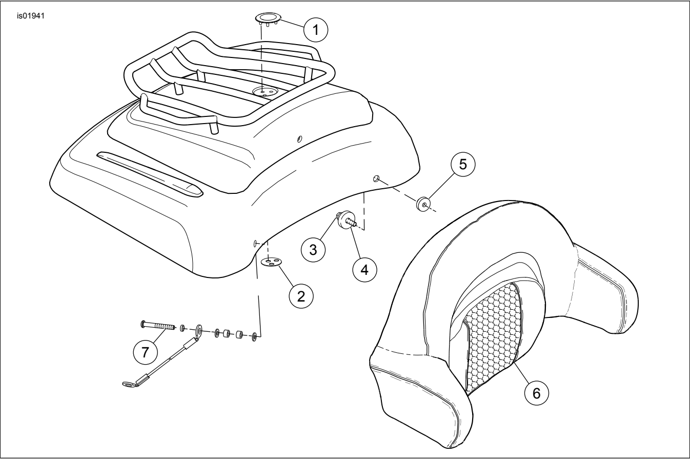
Abbildung 5. Ersatzteile für den Tour-Pak-Einbauteilesatz (oberer Teil)
