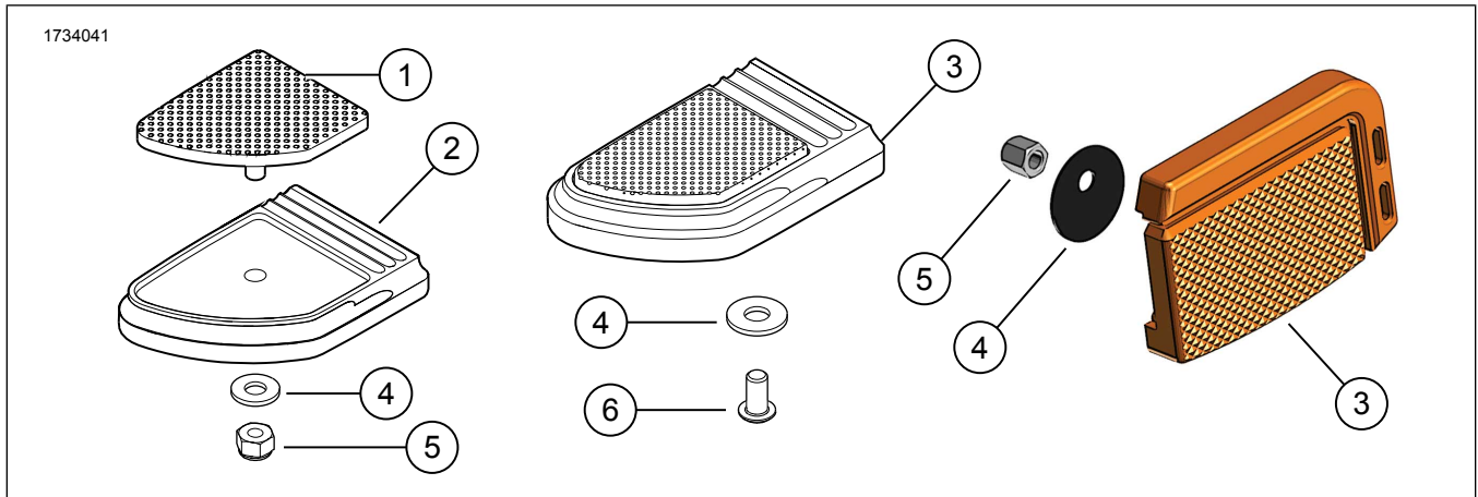
รูปภาพ 1 เนื้อหาเกี่ยวกับชุดอุปกรณ์: ชุดแป้นเหยียบเบรก
