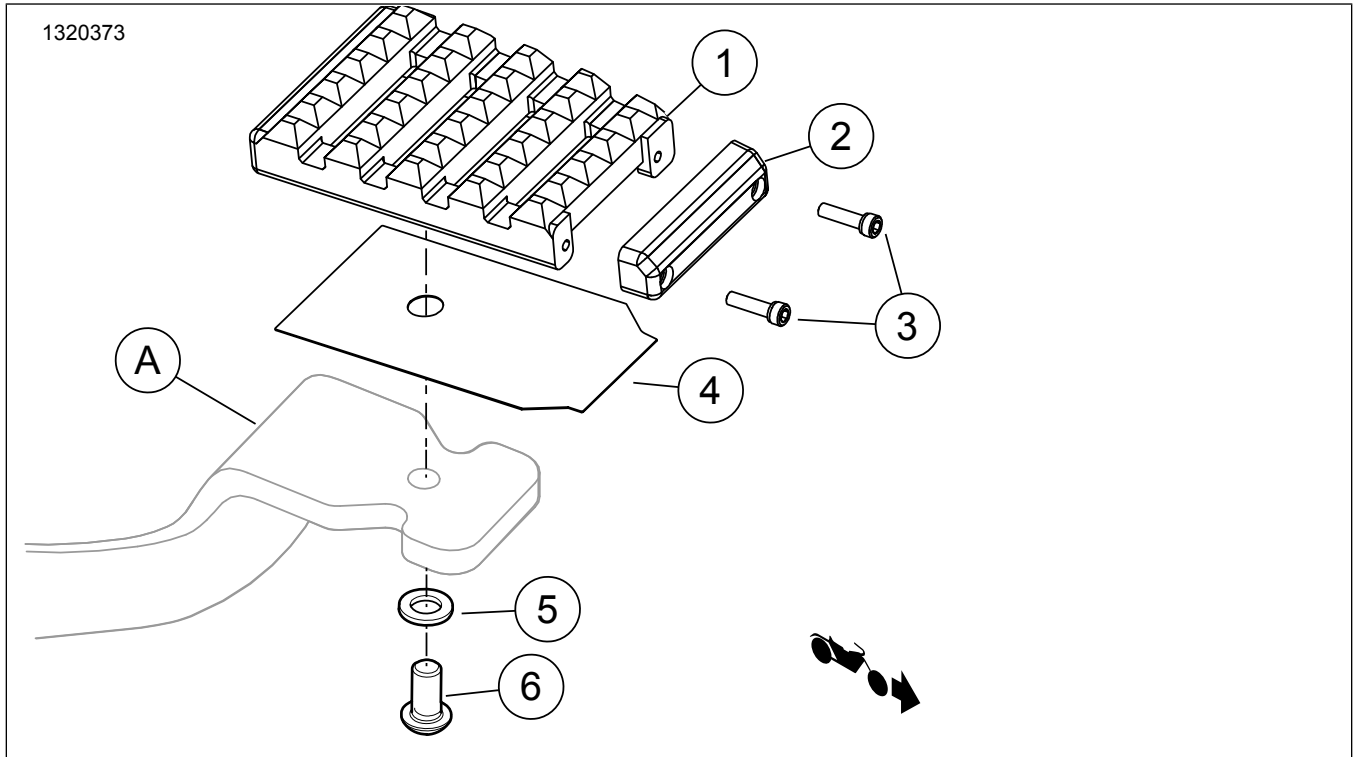
รูปภาพ 1 เนื้อหาเกี่ยวกับชุดอุปกรณ์: ส่วนประกอบชุดแป้นเหยียบเบรก
