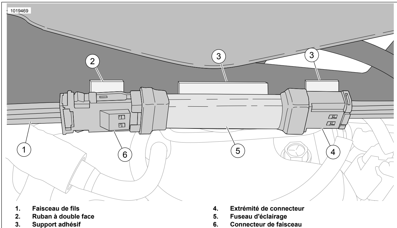
Figure 1. Fuseau d'éclairage, connecteurs et ruban à double face
