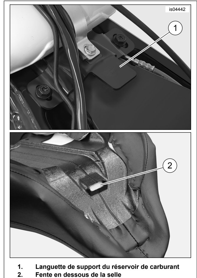
Figure 1. Support de montage avant de la selle
