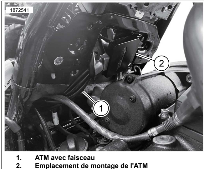
Figure 5. Emplacement de montage de l'ATM
