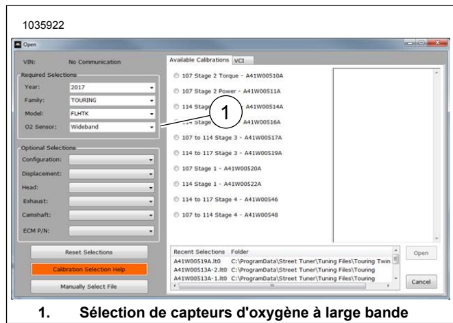
Figure 45. Sélection de capteurs d'oxygène à large bande
