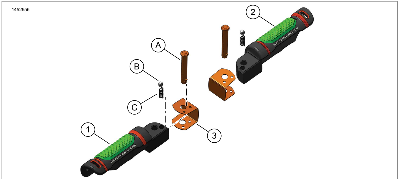
Figure 1. Contenu du kit : Appuie-pied - Passager
