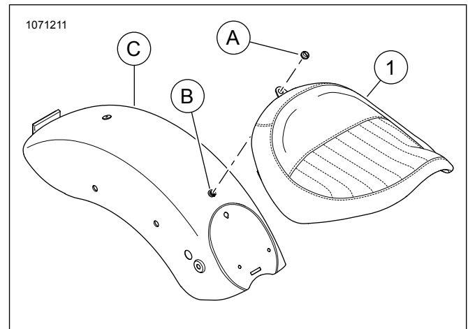
Figure 1. Pièces de rechange : Support de montant simple
