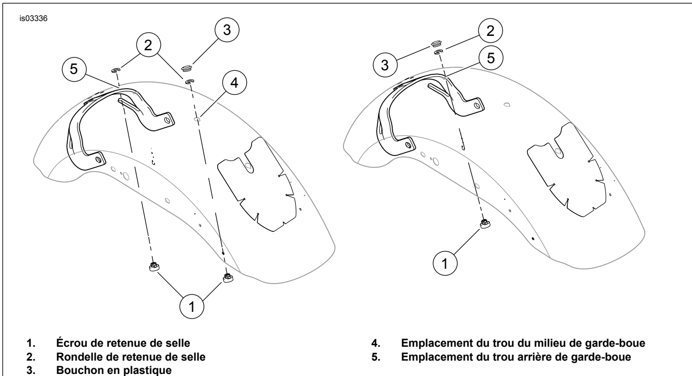
Figure 2. Emplacements de l'écrou et de la rondelle de retenue de la selle
