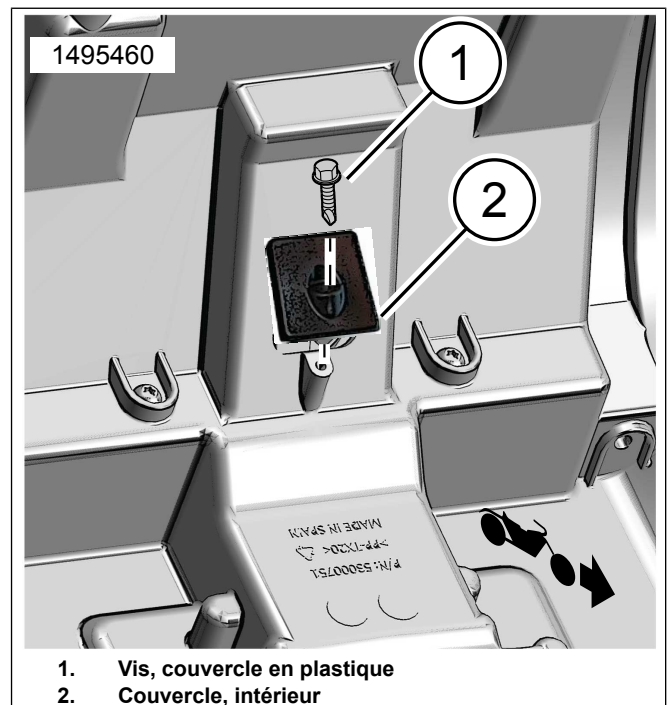
Figure 10. Installation intérieure du couvercle
