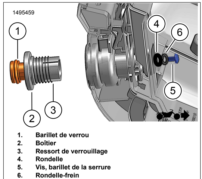
Figure 9. Installer le serrure sur le Top Case
