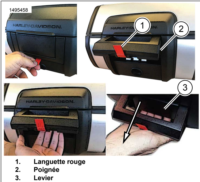
Figure 2. Ouvrir le Top Case
