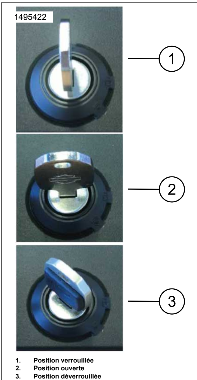
Figure 11. Positions de verrouillage (typiques)
