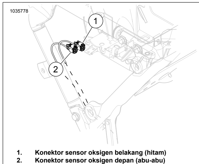
Gambar 10. Lokasi Sensor Oksigen Depan dan Belakang
