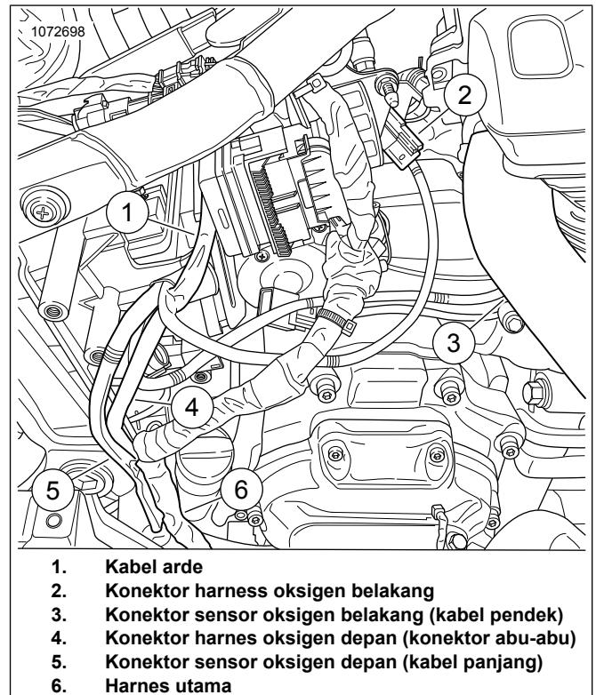
Gambar 24. Pengaturan Jalur Harness ATM
