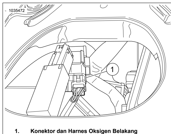
Gambar 38. Lokasi Sensor Oksigen Belakang
