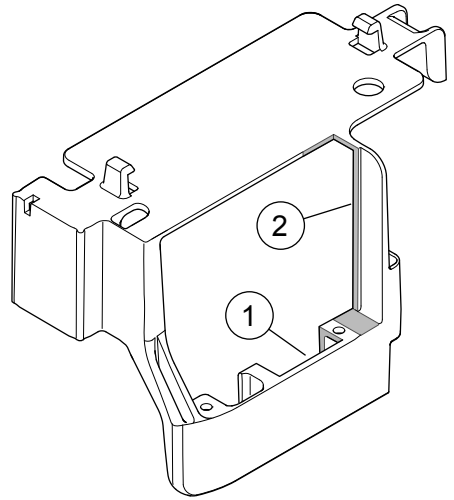
Gambar 30. Tampak Belakang, Caddy yang Dipotong
