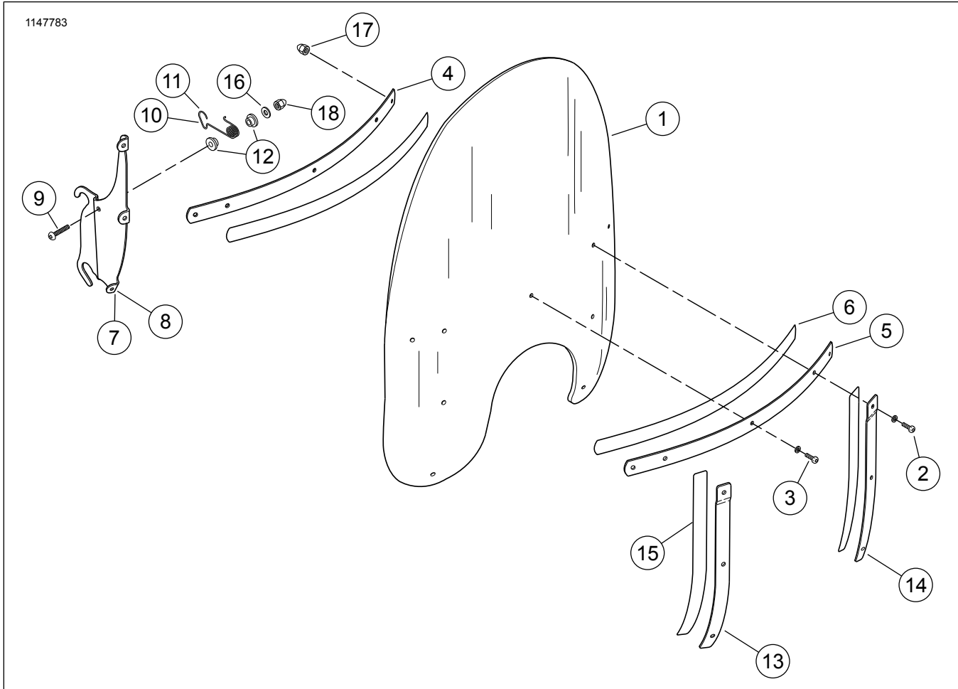
Gambar 1. Komponen Servis: Unit Kaca Depan
