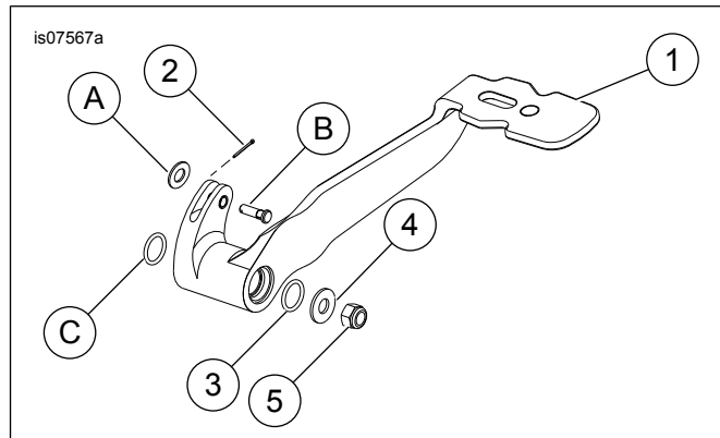
Gambar 1. Komponen Servis: Tuas Rem Belakang (Tipikal Ditampilkan)
