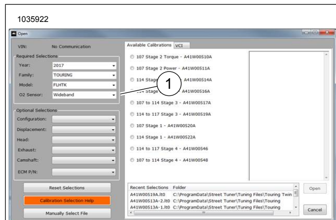
1. Volba širokopásmové lambda sondy
