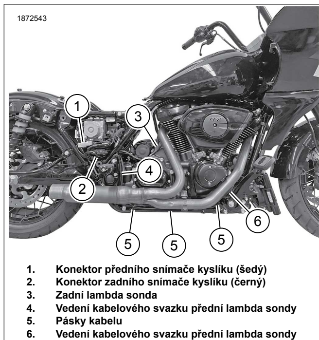
Ilustrace 8. Vedení kabelov'ho svazku snímače modulu ATM
