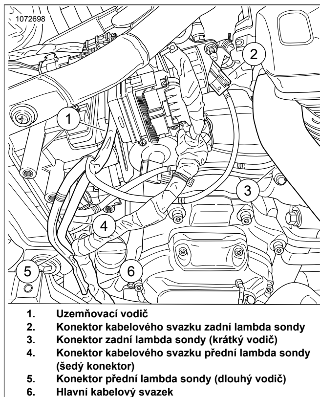
Ilustrace 24. Vedení kabelového svazku modulu ATM
