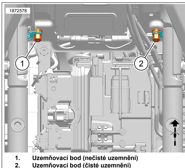
Ilustrace 7. Umístění uzemňovacích bodů skříně akumulátoru
