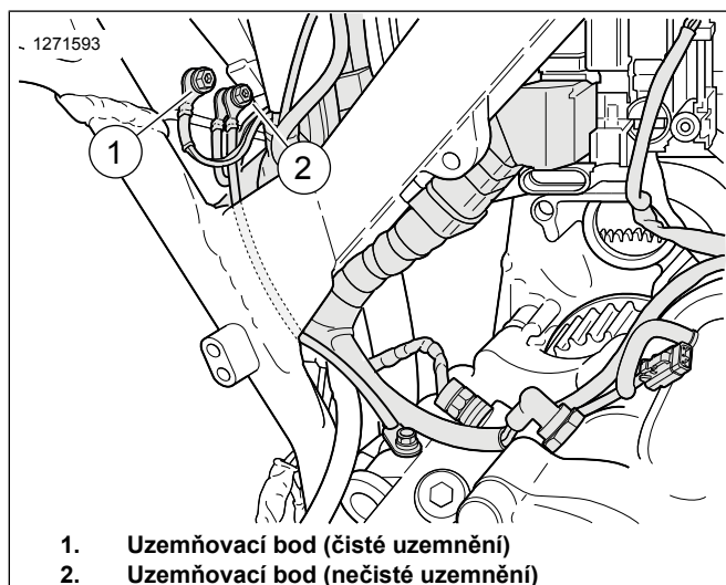
Ilustrace 42. Umístění uzemňovacích bodů skřínky akumulátoru
