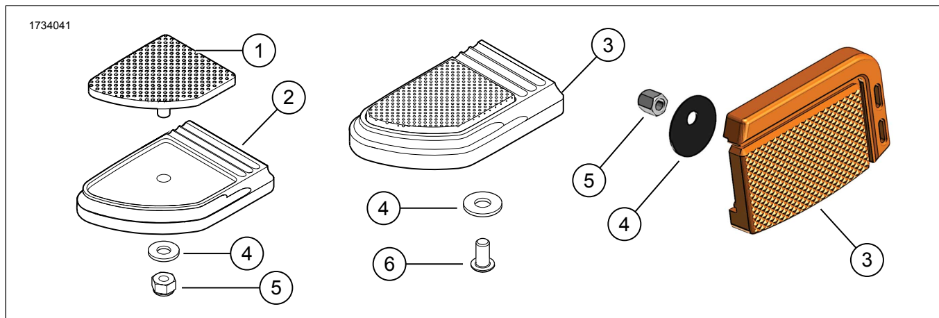
Ilustrace 1. Obsah sady: Sada krytky brzdového pedálu
