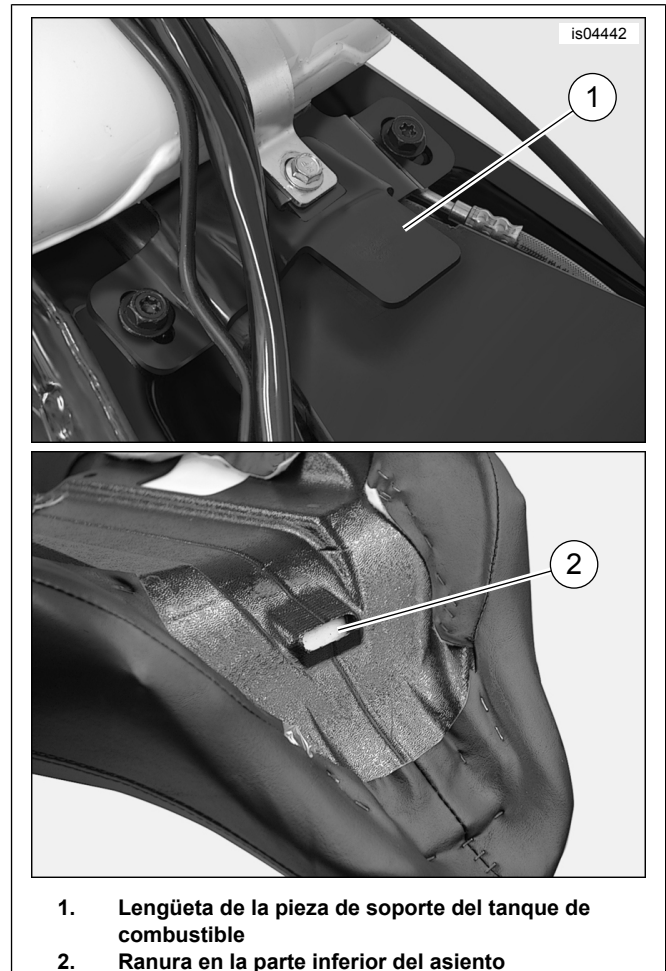
Figura 1. Montaje del asiento delantero
