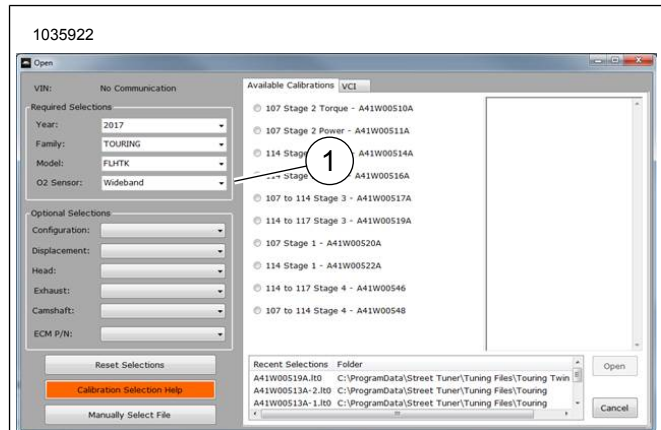
Figura 45. Selección del sensor de oxígeno de banda ancha
