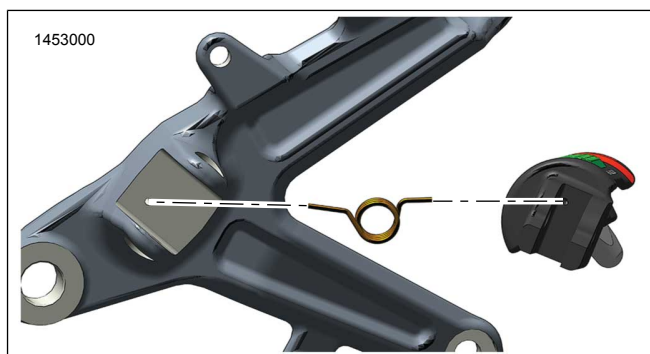
Figura 5. Orientación del resorte de retorno - lado derecho
