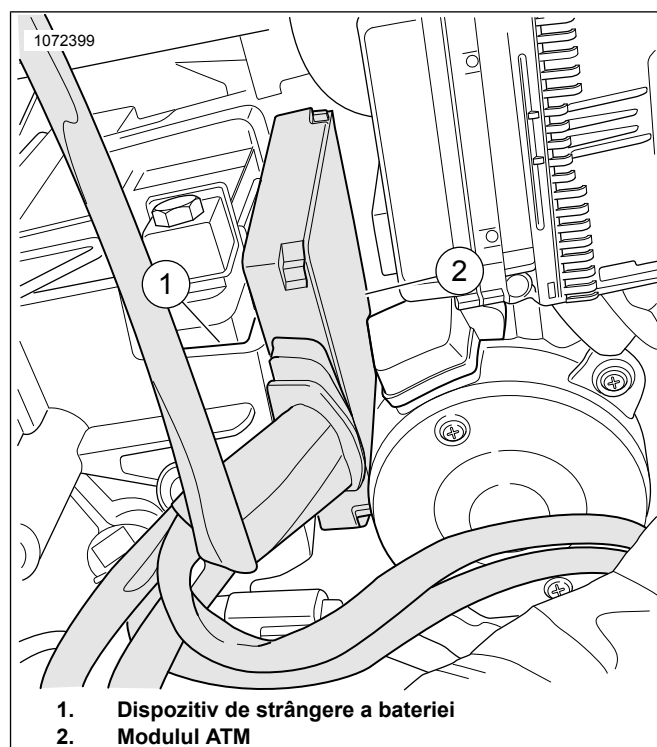
Figura 18. Plasați modulul
