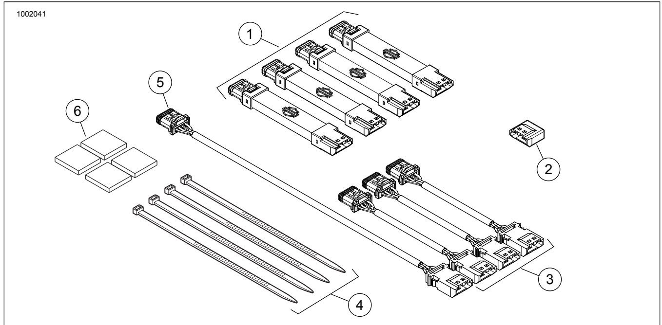
Figure 2. Mga Pamalit na Piyesa, Mga Spectra Glo Light Pod Kit
