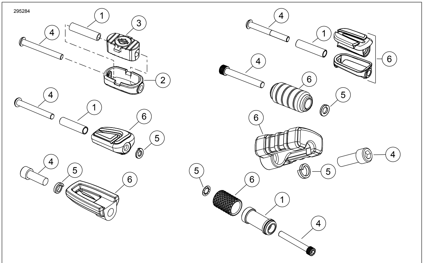
Figure 1. Mga Nilalaman ng Kit: Shifter Peg Kit
