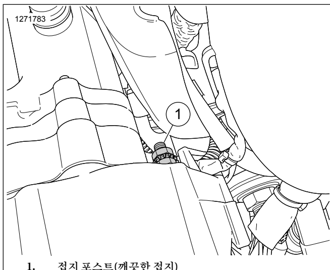
그림 49. Sportster 접지
