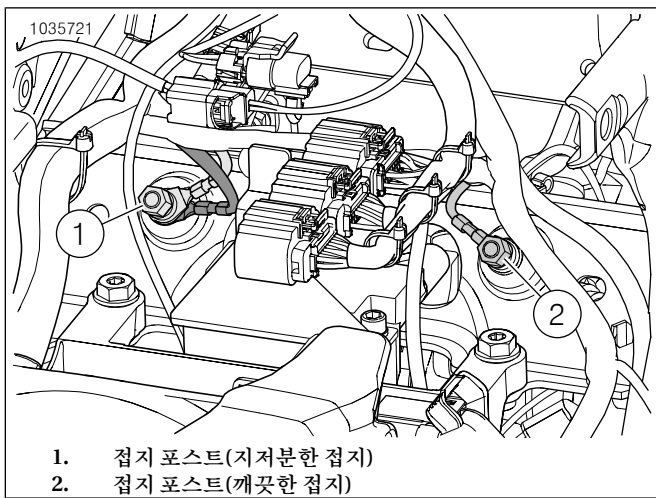
그림 15. 배터리 박스 접지 포트 위치
