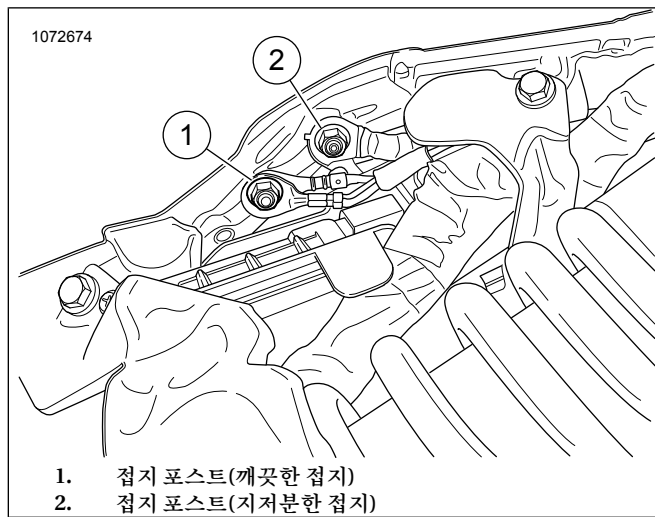
그림 23. 프레임 접지
