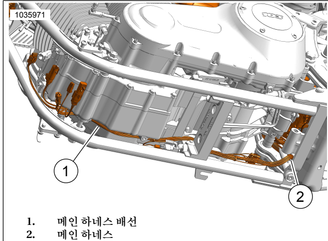
그림 36. 하네스 배선
