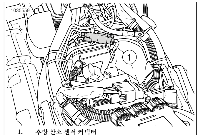
그림 31. 후방 산소 센서 위치
