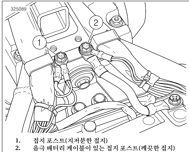
그림 34. 배터리 박스 접지 포스트 위치
