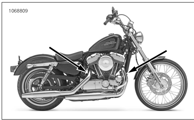
그림 48. 산소 센서 위치(배기 파이프의 안쪽 측면)
