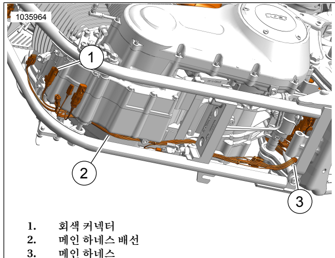
그림 35. 하네스 배선
