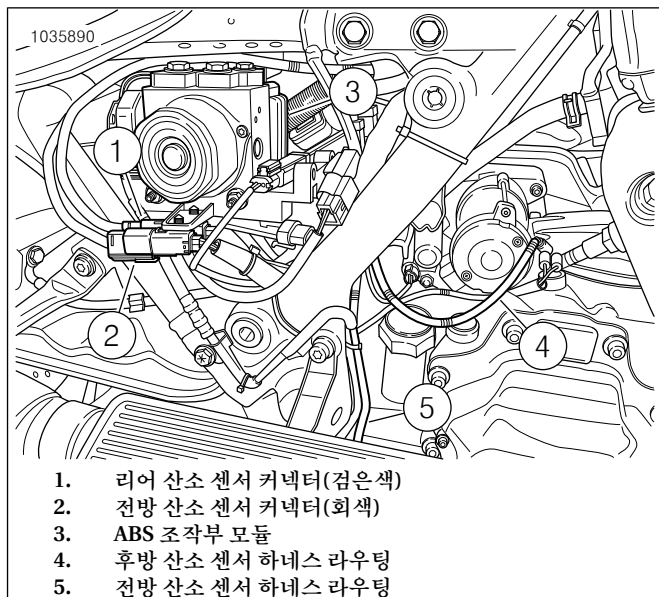
그림 16. ATM 센서 하네스 배선
