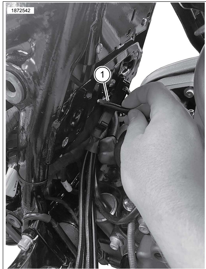
그림 6. 접지선 라우팅
