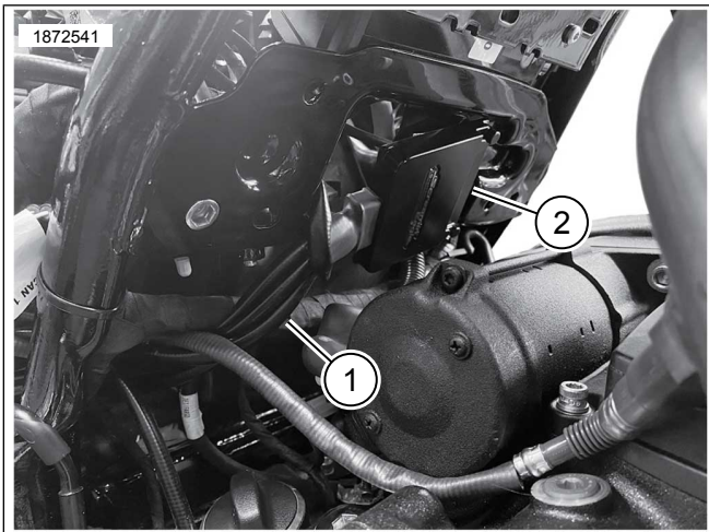
그림 5. ATM 장착 위치
