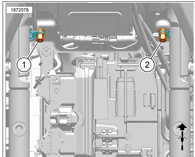
그림 6. 접지선 라우팅
