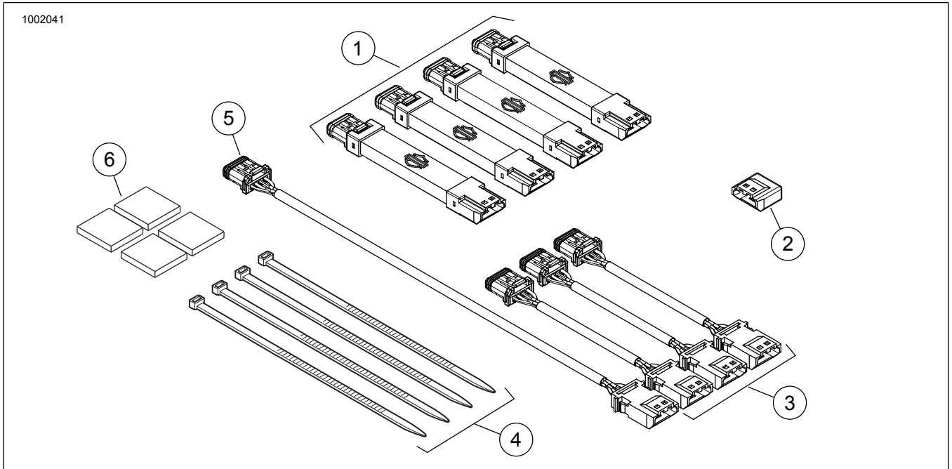
그림 2. 정비 부품, Spectra Glo 라이트 포트 키트
