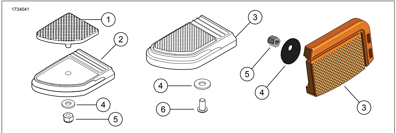
그림 1. 키트 내용물: 브레이크 페달 패드 키트
