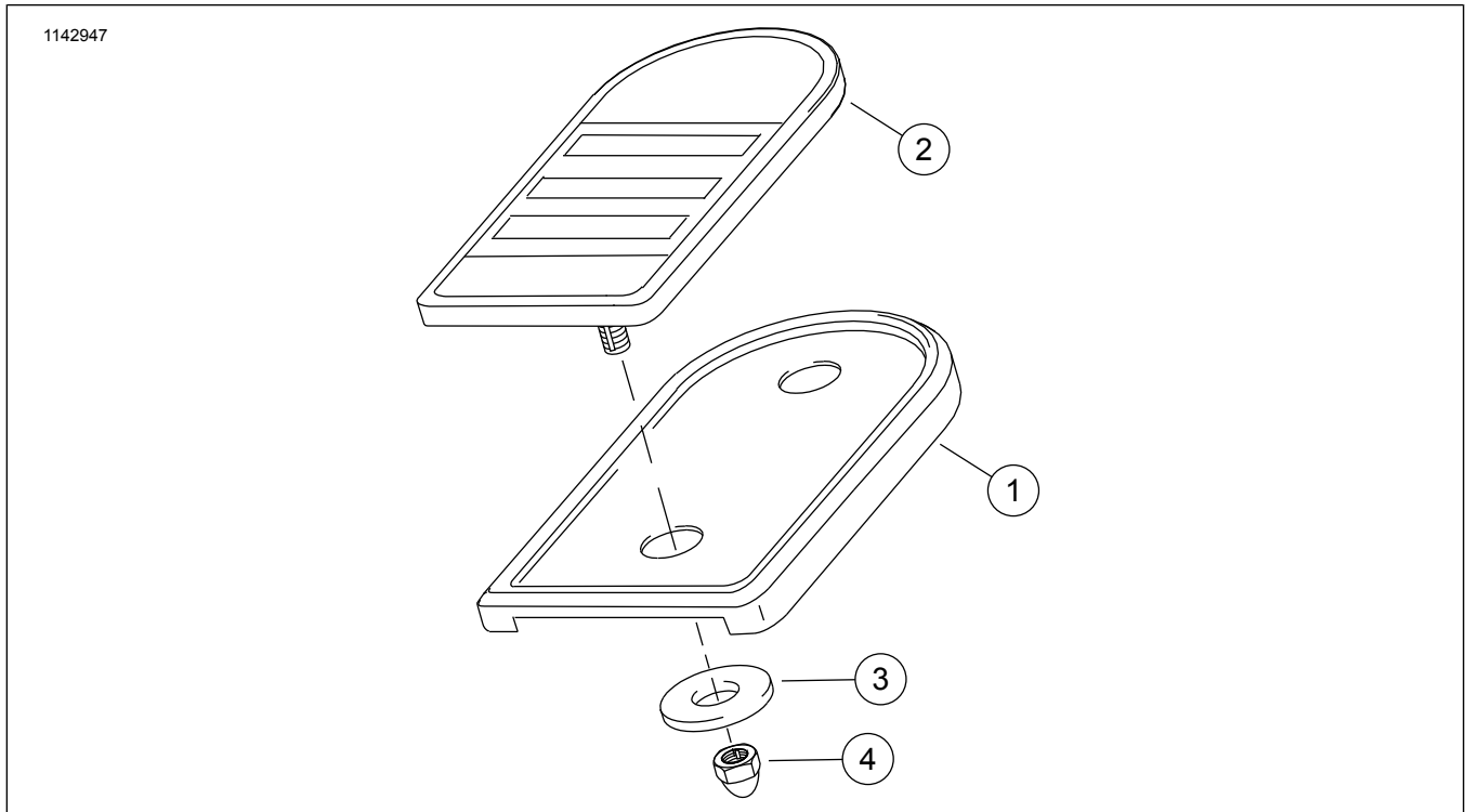
圖1。套件內容：鍍鉻煞車踏板墊工具包-大型部件
