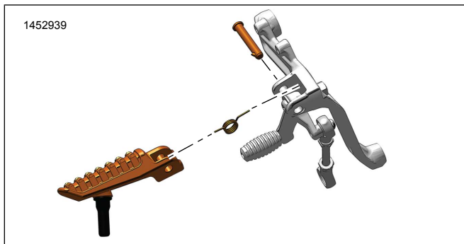
圖4。腳樁-騎士-左側
