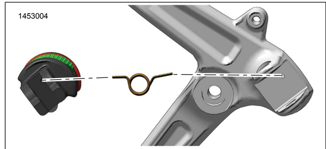
圖6。回彈彈簧方向-左側
