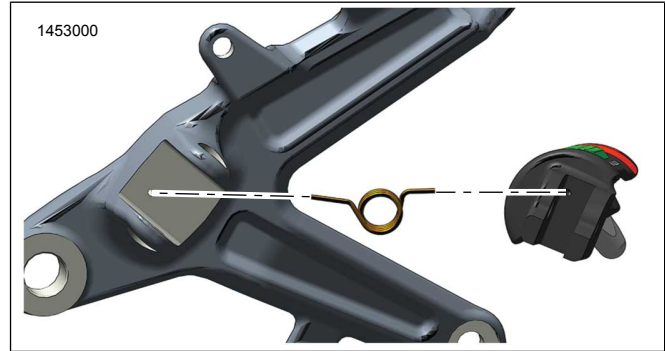
圖5。回彈彈簧方向-右側
