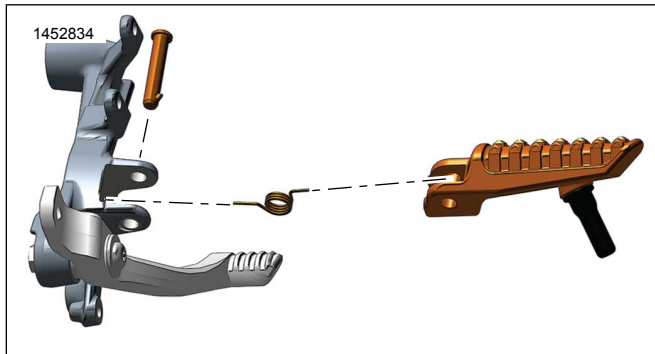
圖3。腳樁-騎士-右側
