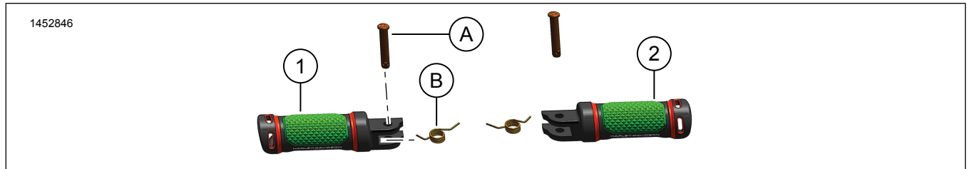
圖1。套件內容：競品腳樁 - 騎士
