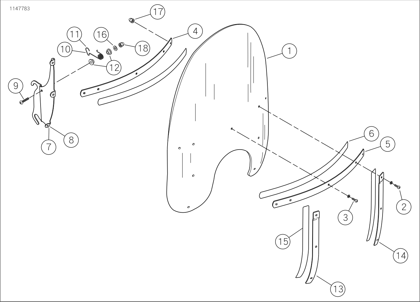
圖1。維修零件擋風玻璃組件
