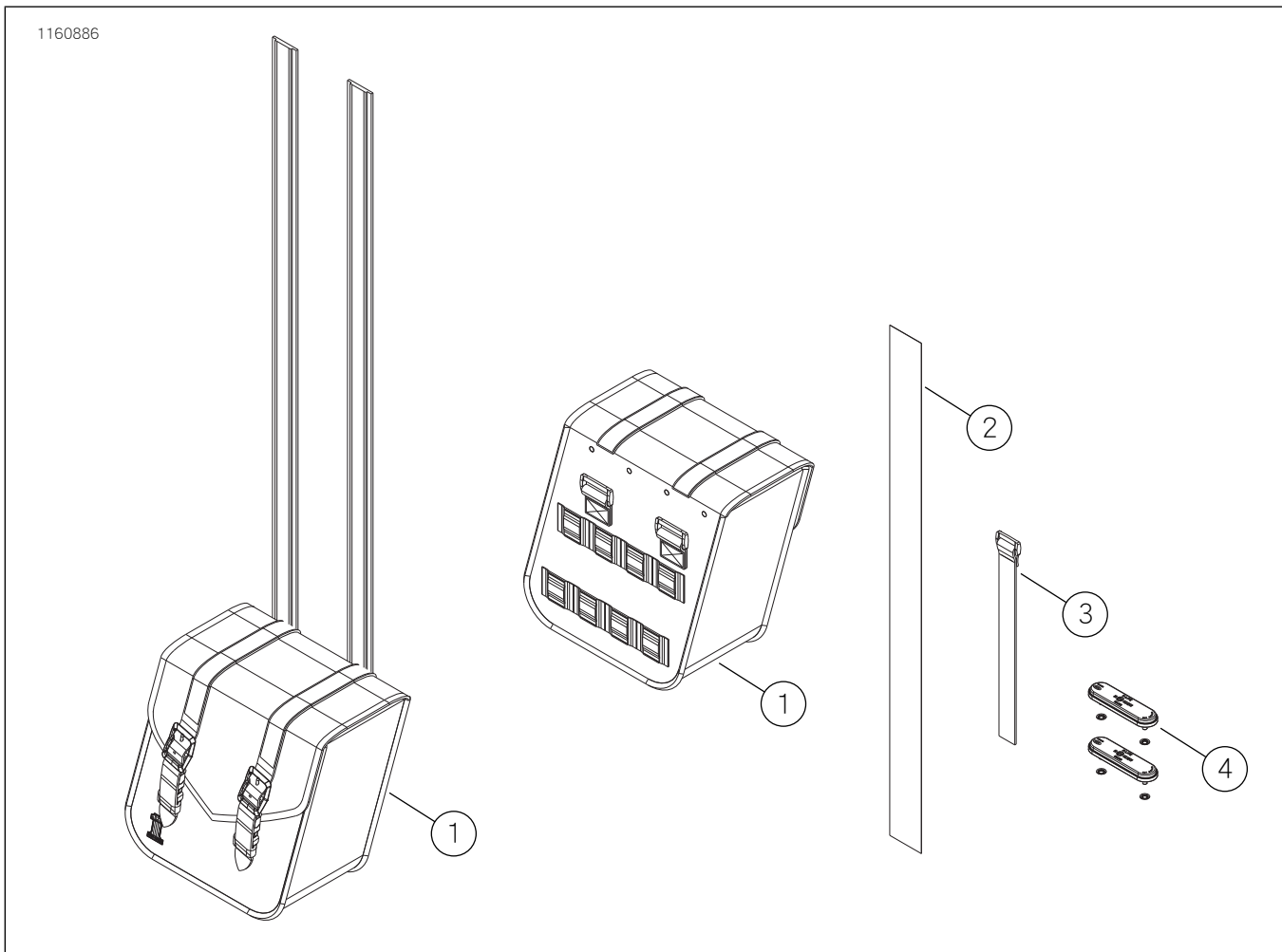
圖4。維修零件：轉換側箱套件（顯示精簡版）
