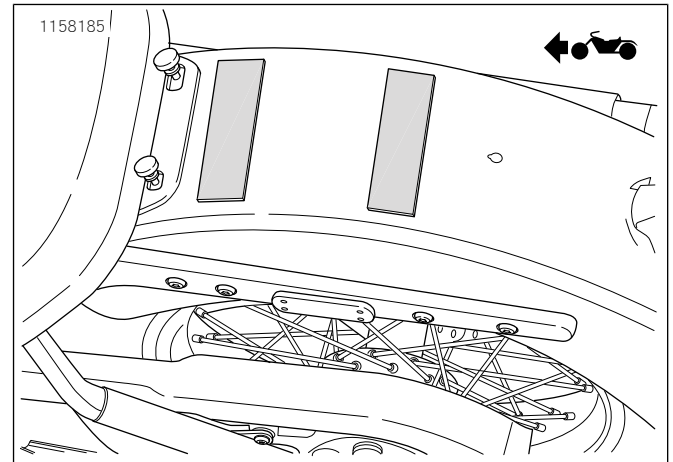
圖1. 防磨擦帶放置
