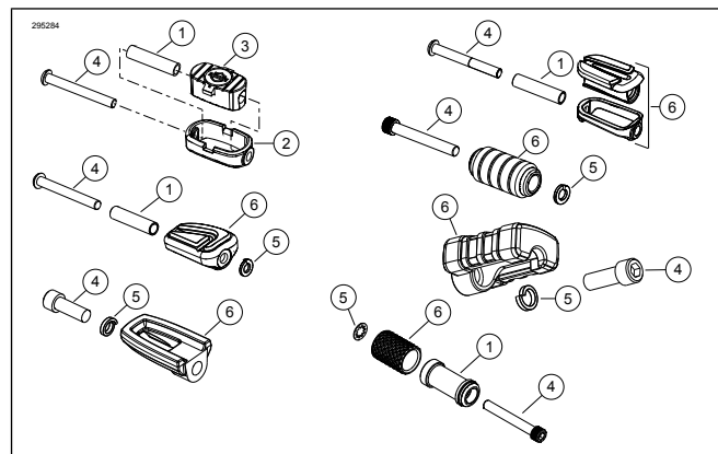
Figura 1. Kit de pedal do câmbio
