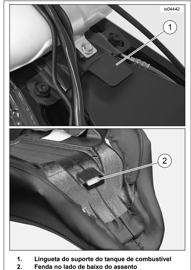
Figura 1. Montagem dianteira do assento
