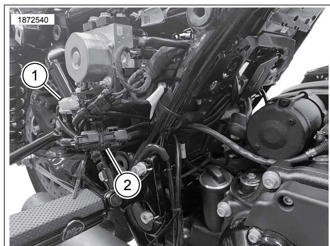
Figura 4. Conexões do chicote de fios principal do ATM
