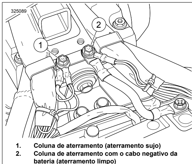
Figura 34. Localizações da coluna de aterramento na caixa de bateria
