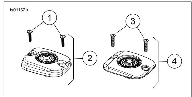
Figura 1. Peças de reposição: Kits de tampa do cilindro-mestre
