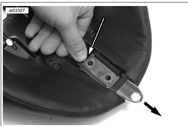
Figura 1. Remoção do suporte do assento (Suporte de retenção mostrado)
