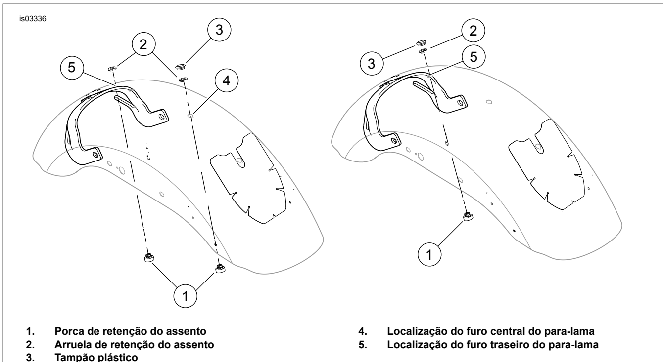
Figura 2. Localização da porca de retenção e da arruela do assento
