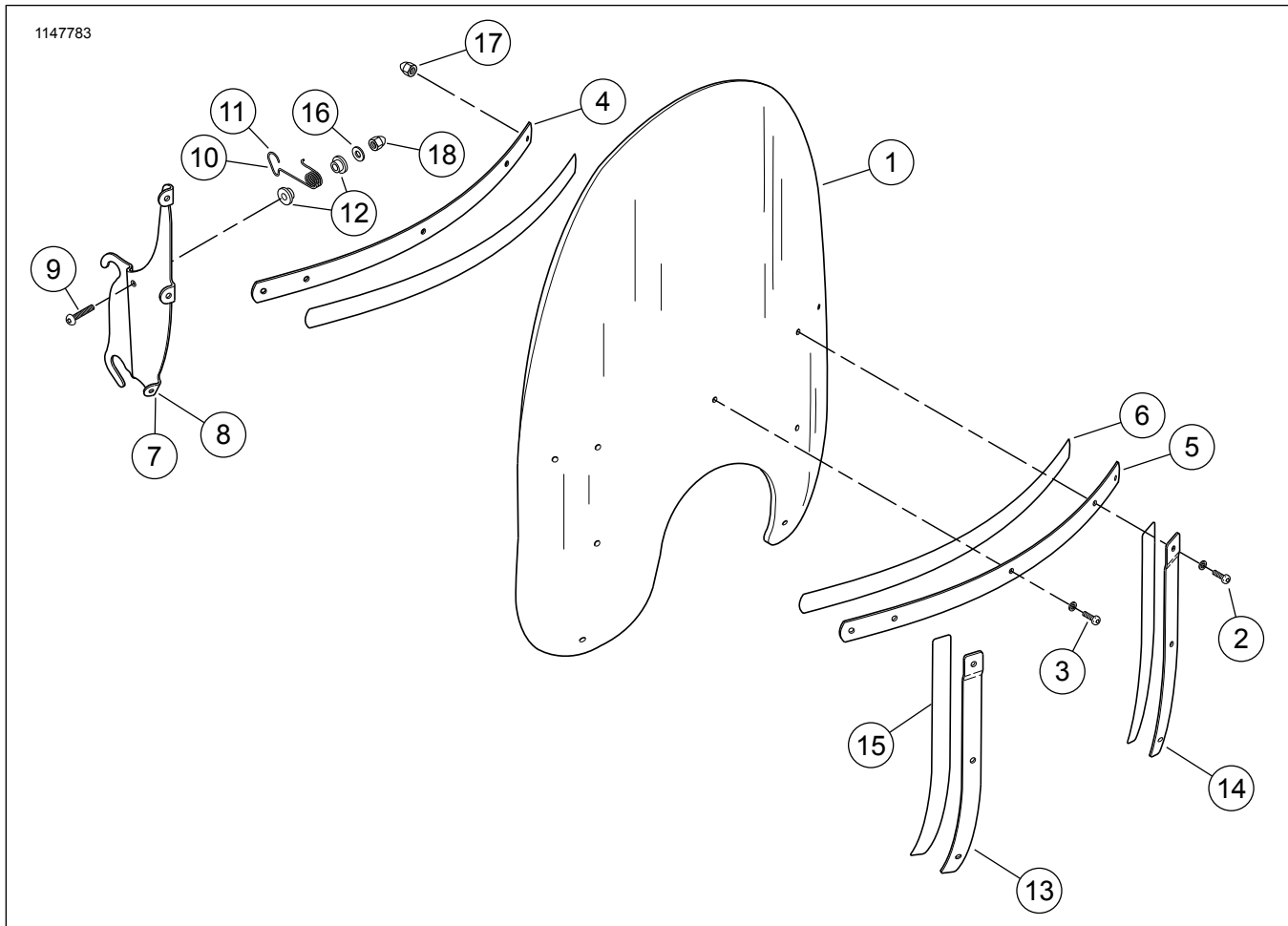
Figura 1. Peças de reposição: Montagem do pára-brisa
