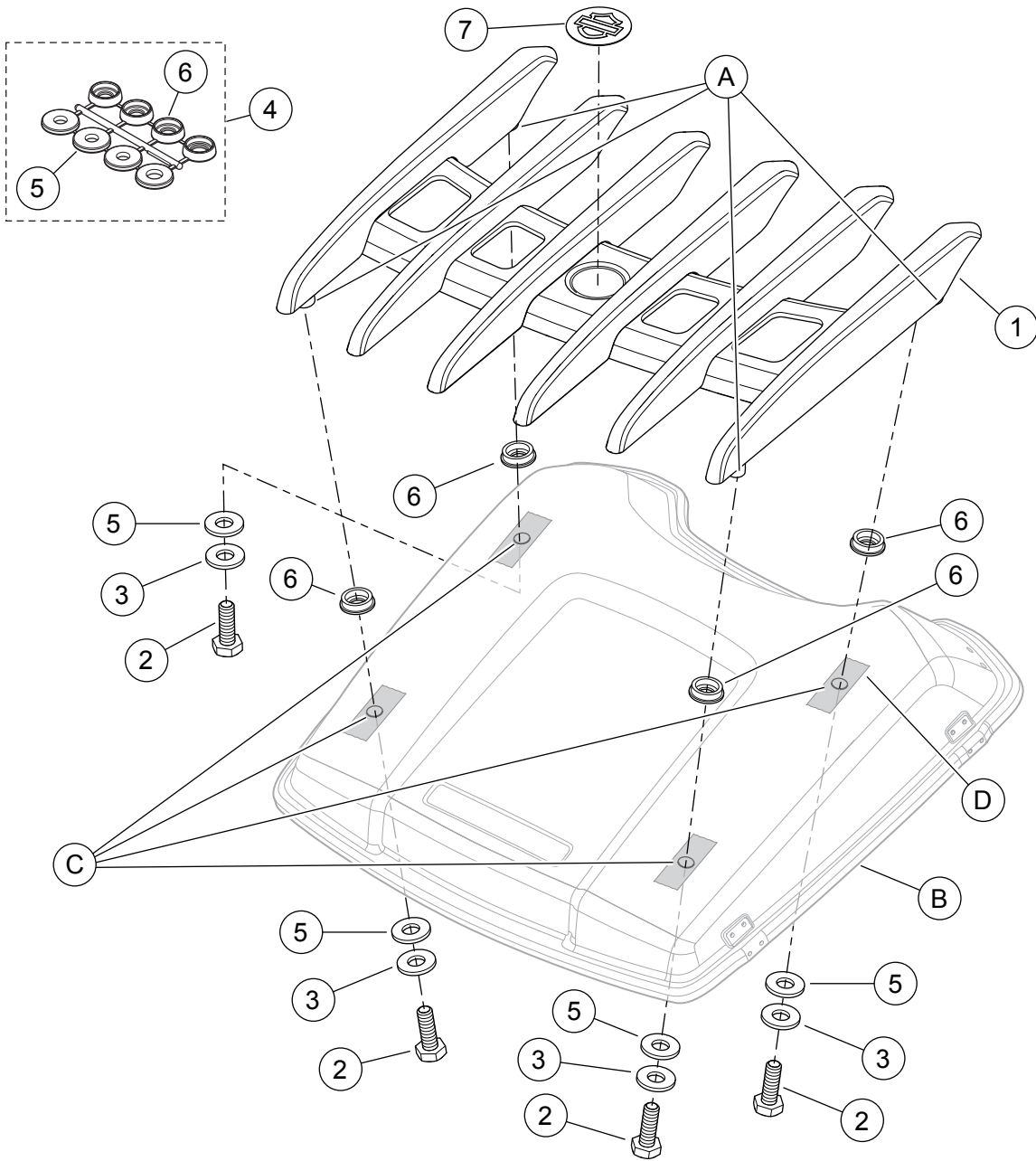
Figura 1. Peças de reposição, kit de bagageiro Tour-Pak Stealth
