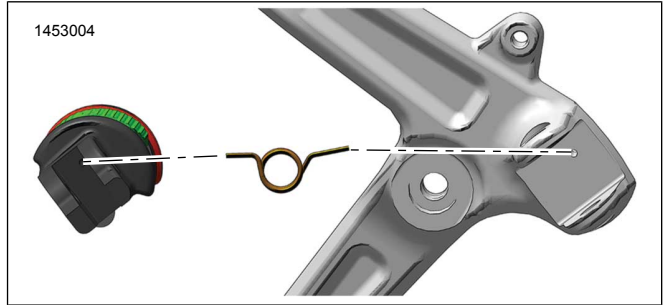
Şekil 6. Geri Çekme Yayının Yönü - Sol
