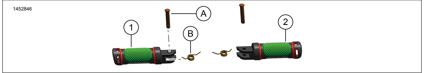
Şekil 1. Kit İçerikleri: Adversary Ayaklıklar - Sürücü
