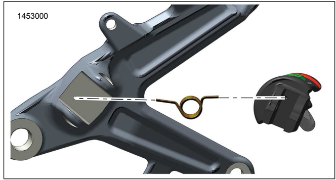
Şekil 5. Geri Çekme Yayının Yönü - Sağ
