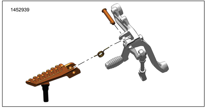
Şekil 4. Ayaklık - Sürücü - Sol
