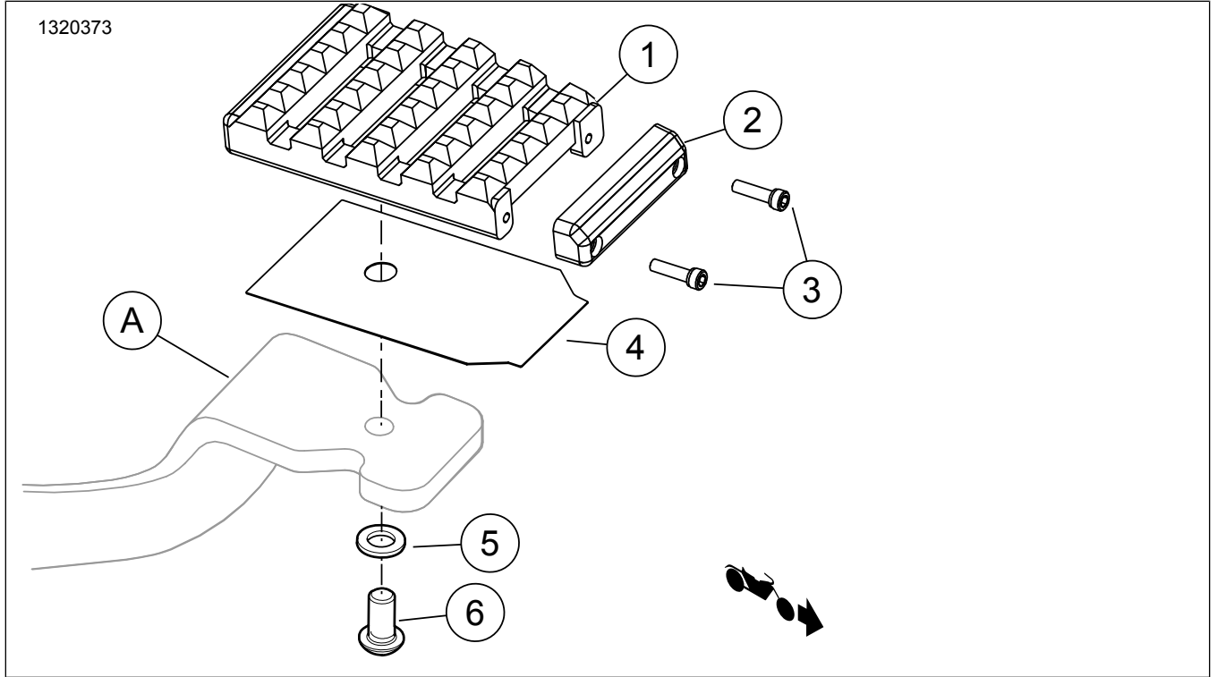
Şekil 1. Kit İçerikleri: Fren Pedal Yastığı Bileşenleri
