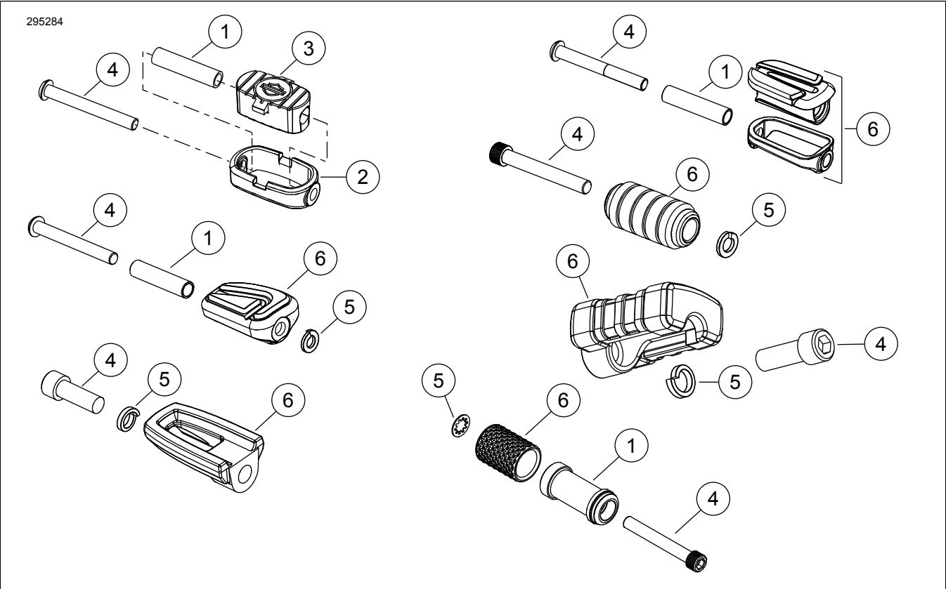
Rajah 1. Kit Pancang Penganjak
