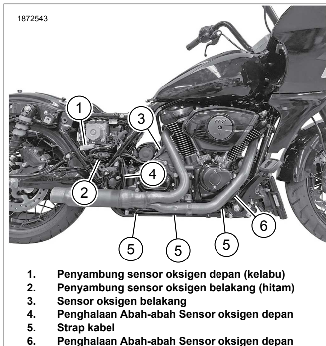
Rajah 8. Penghalauan Abah-abah Sensor ATM
