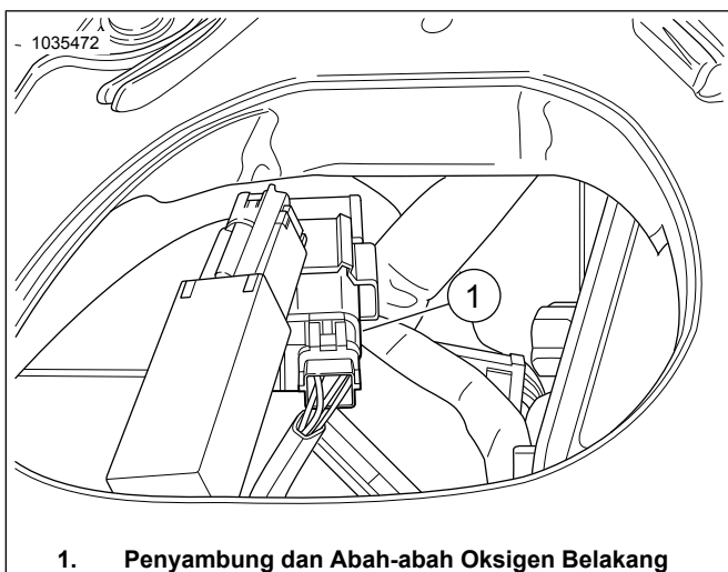
1. Penyambung dan Abah-abah Oksigen Belakang Rajah 38. Lokasi Sensor Oksigen Belakang
