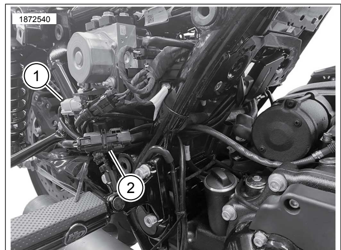
Rajah 4. Sambungan Abah-abah Utama ATM
