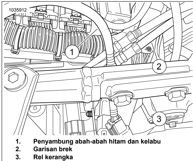
Rajah 12. Penghalaan Abah-abah Penyambung Kelabu dan Hitam
