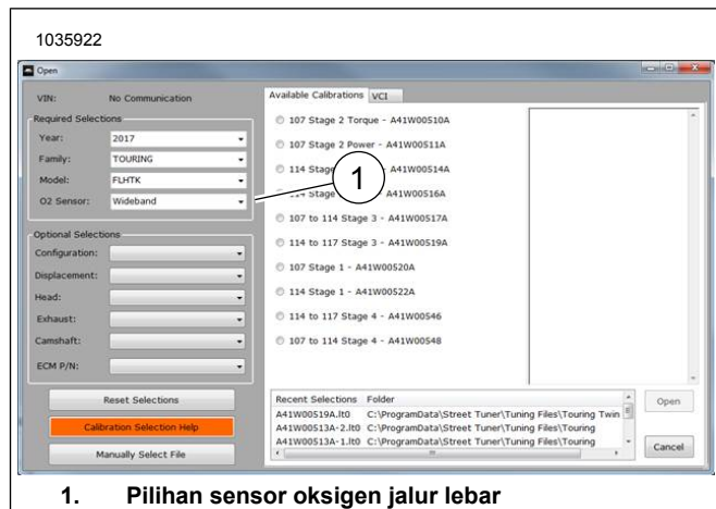
Rajah 45. Pilihan Sensor Oksigen Jalur Lebar
