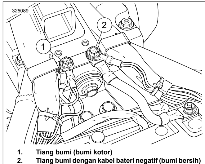
Rajah 34. Lokasi Tiang Bumi Kotak Bateri
