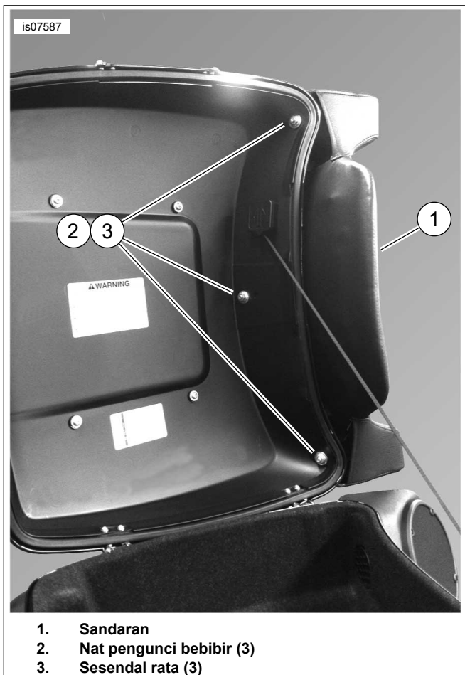
Rajah 1. Sandaran Terlekap pada Penutup King Tour-Pak
