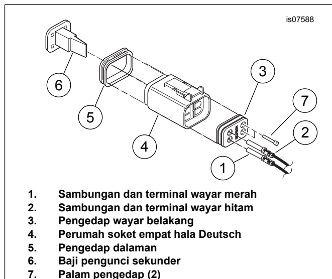
Rajah 2. Masukkan Terminal ke dalam Perumah Soket Deutsch
